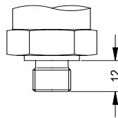
G 1/4" DIN 3852 M 10x1 M 12x1 M 12x1,5
