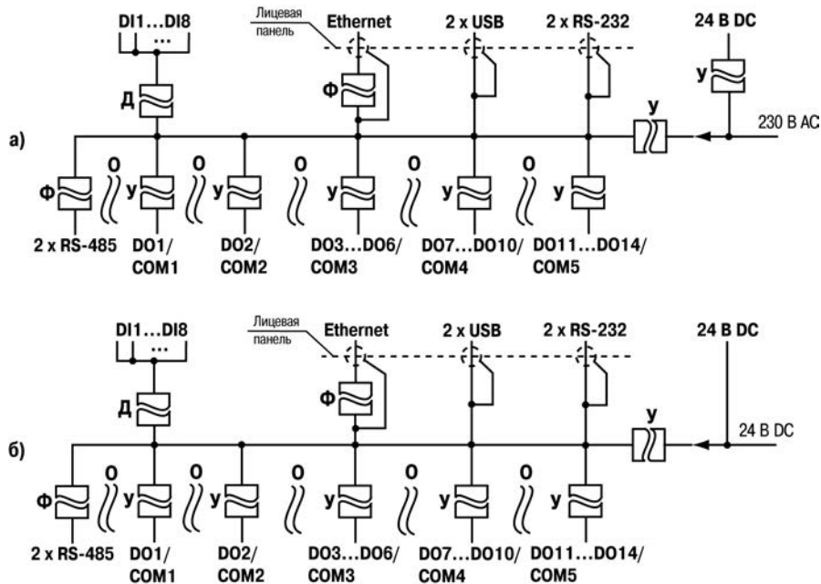
Рисунок 2.1 – Схема электрической прочности изоляции ПЛК110-220.х.Р (а) и ПЛК110-24.х.Р (б)
