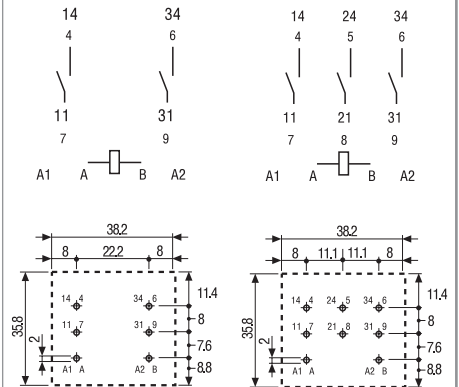
62.22 - 0300 Вид сбоку
