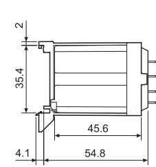
062.07 с реле
