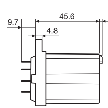
062.10 с реле
