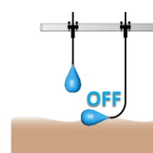
Le niveau mini arrête la pompe
