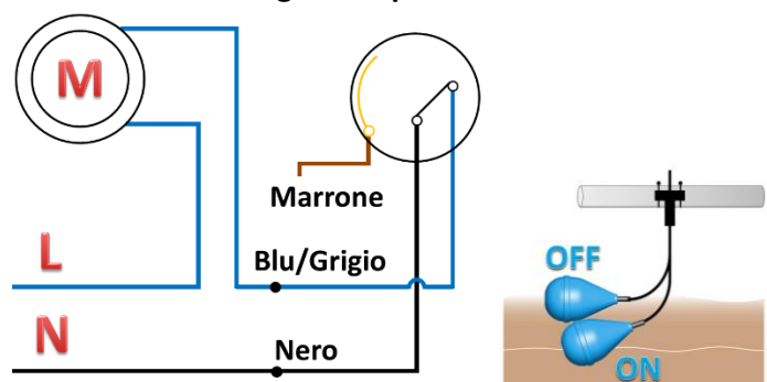
Fig.3 riempimento
