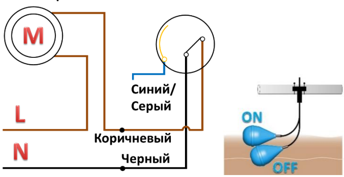
Рис.2 опорожнение см.
