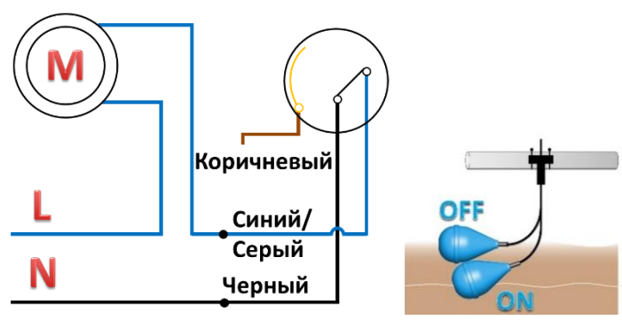
Рис.3 наполнение см.
