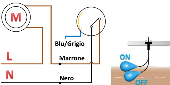
Fig.2 svuotamento
