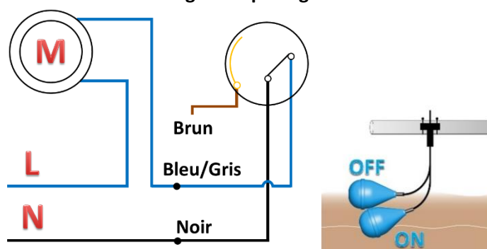
Fig.3 remplissage
